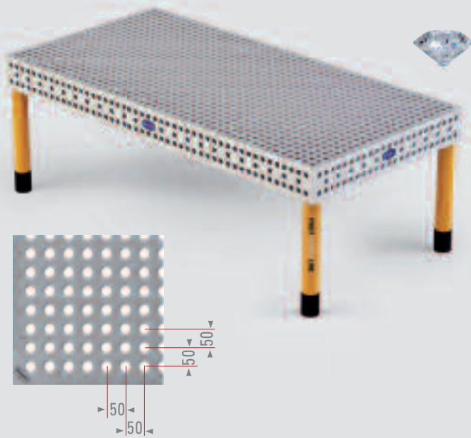
Piastra del tavolo con fori di sistema D28 con griglia da 50 mm x 50 mm
