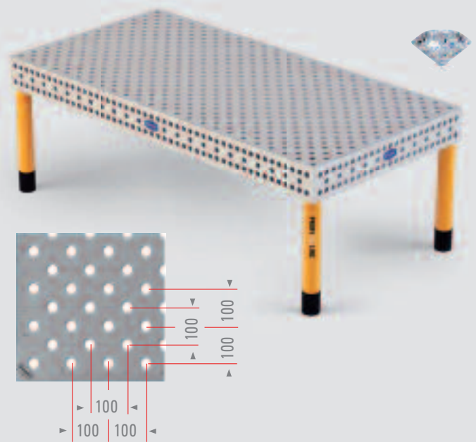
Piastra del tavolo con fori di sistema D28 con griglia diagonale da 100 mm x 100 mm
