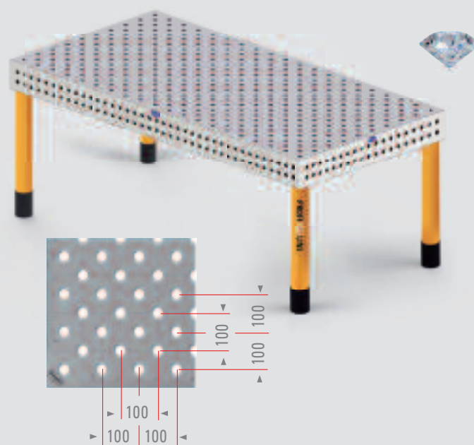
Piastra del tavolo con fori di sistema D22 con griglia diagonale da 100 mm x 100 mm
