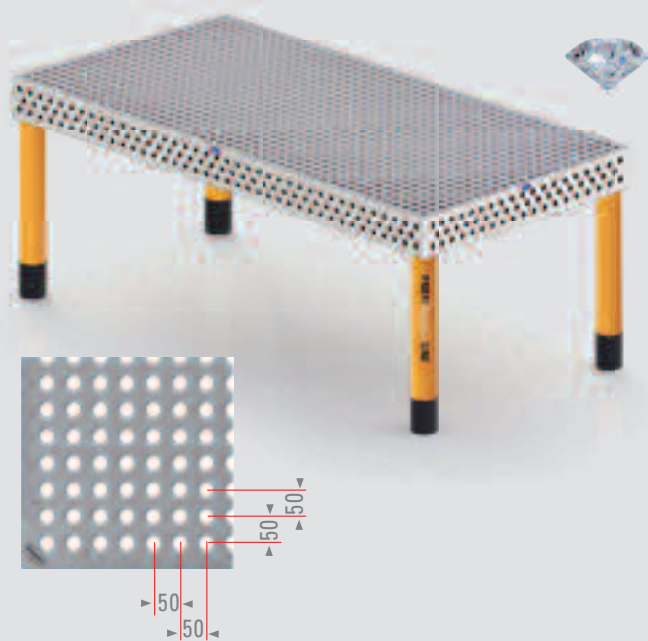
Piastra del tavolo con fori di sistema D22 con griglia da 50 mm x 50 mm
