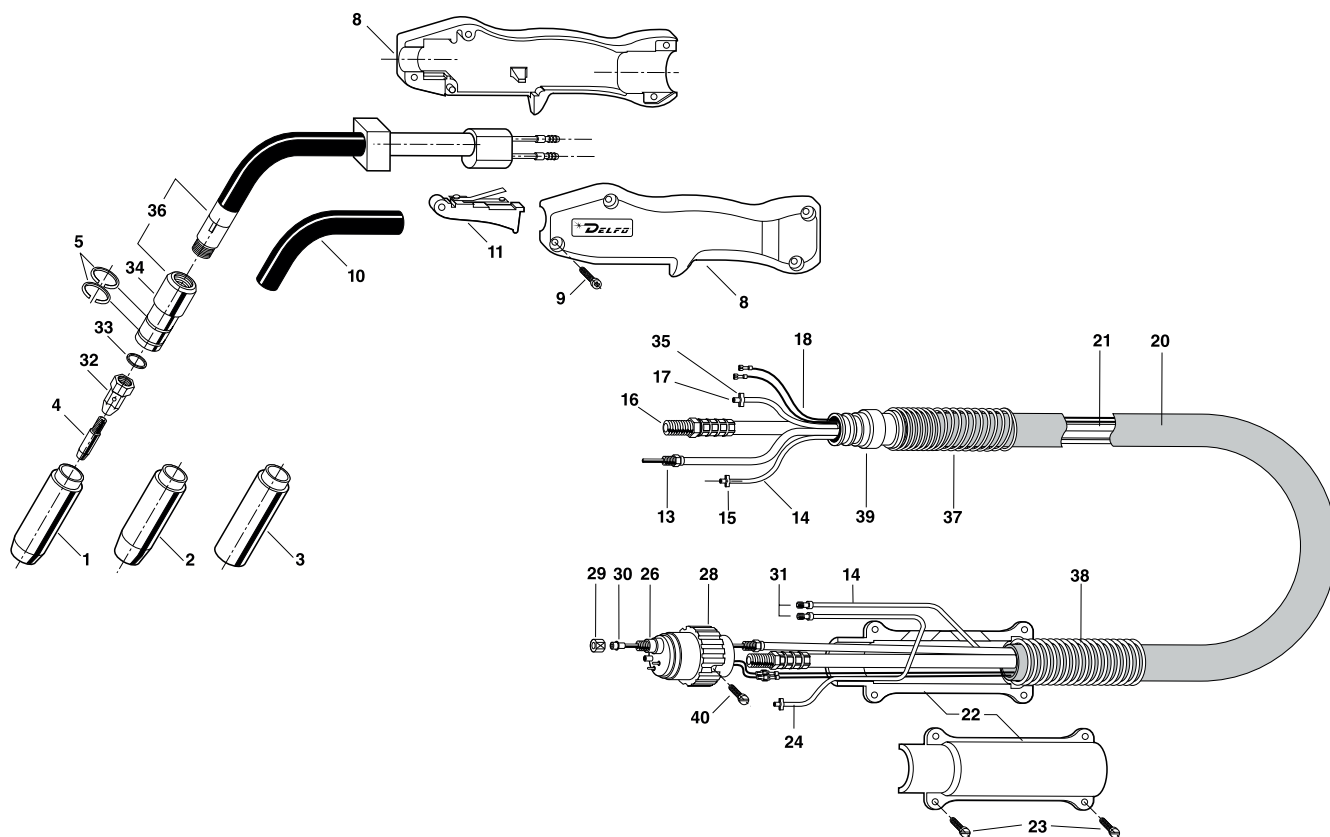
LISTA RICAMBI
