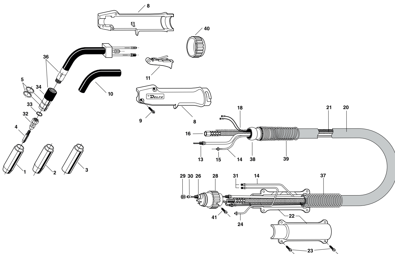
LISTA RICAMBI
