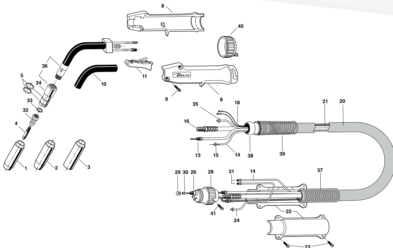
LISTA RICAMBI
