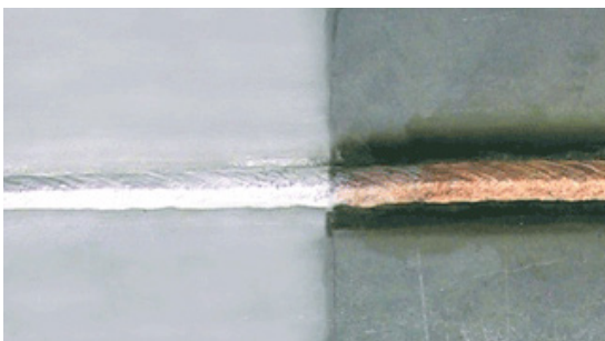
Prima e dopo il decapaggio. Avesta Pickling Paste 101 - per il decapaggio a pennello in tutte le posizioni.
